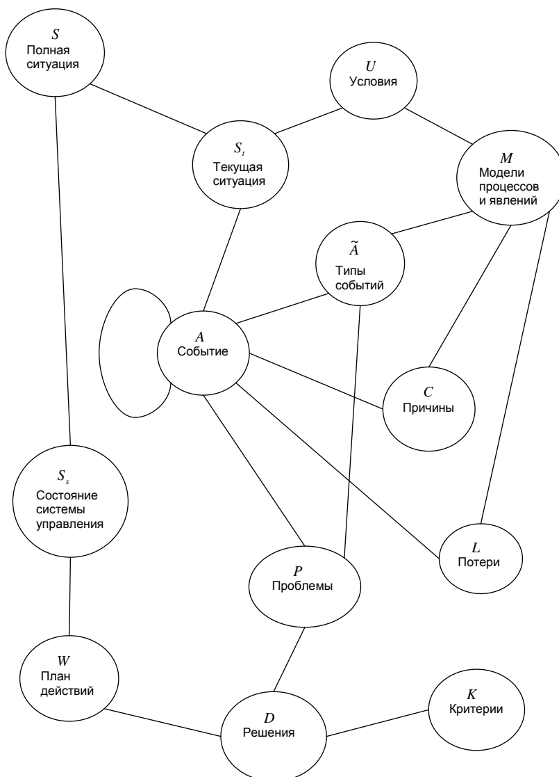
Рис. 2. Диаграмма классов онтологической модели ситуации верхнего уровня
