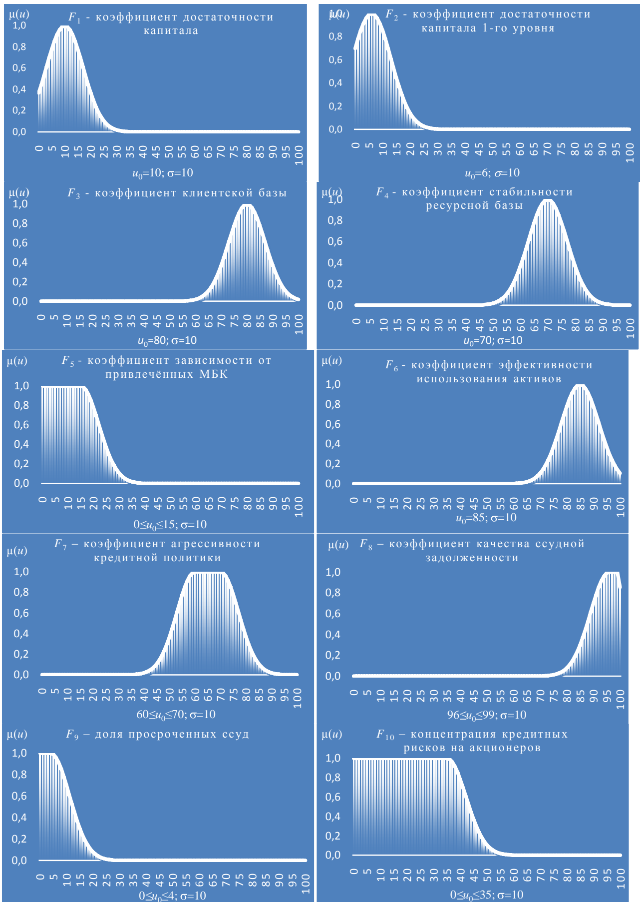
Рис. 1. Функции принадлежности нечетких множеств F_k ( k = 1 \div 10 )
